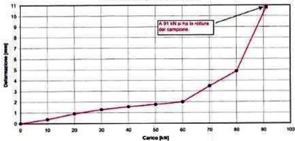
Diagramma carico-deformazione
