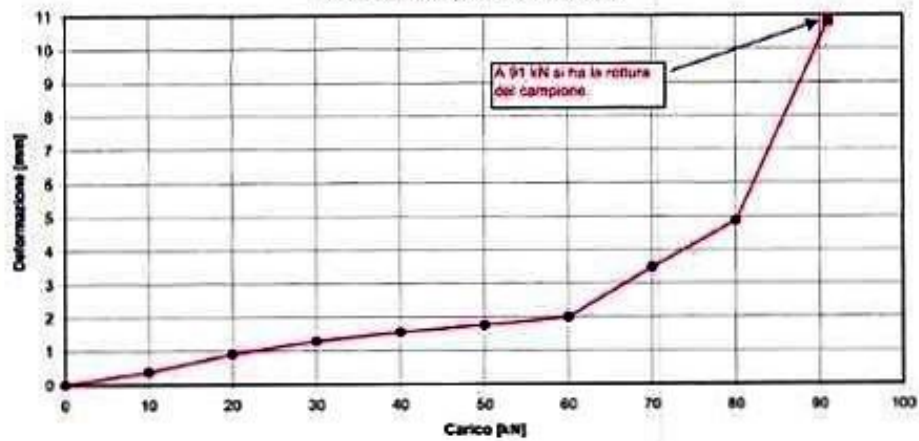
Diagramma carico-deformazione.
