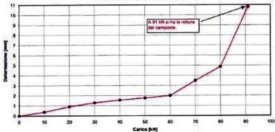
Diagramma carico-deformazione.
