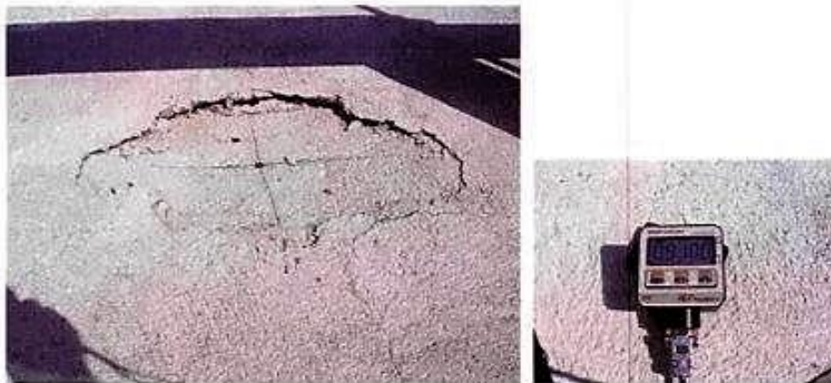
Particolare dell'elemento collassato in mezzeria e della lettura del carico massimo.
